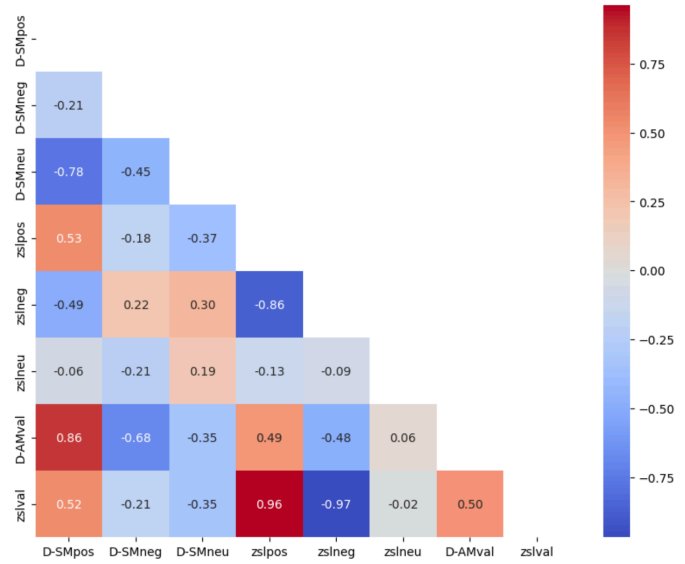
Figure 3.6 – Matrice de corrélations des probabilités de traits.
