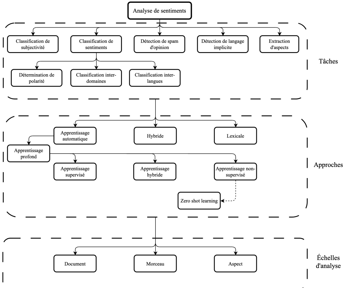
Figure 3.1 – Aperçu du concept d'analyse de sentiments (inspiré de Ligthart et al. (2021)).
