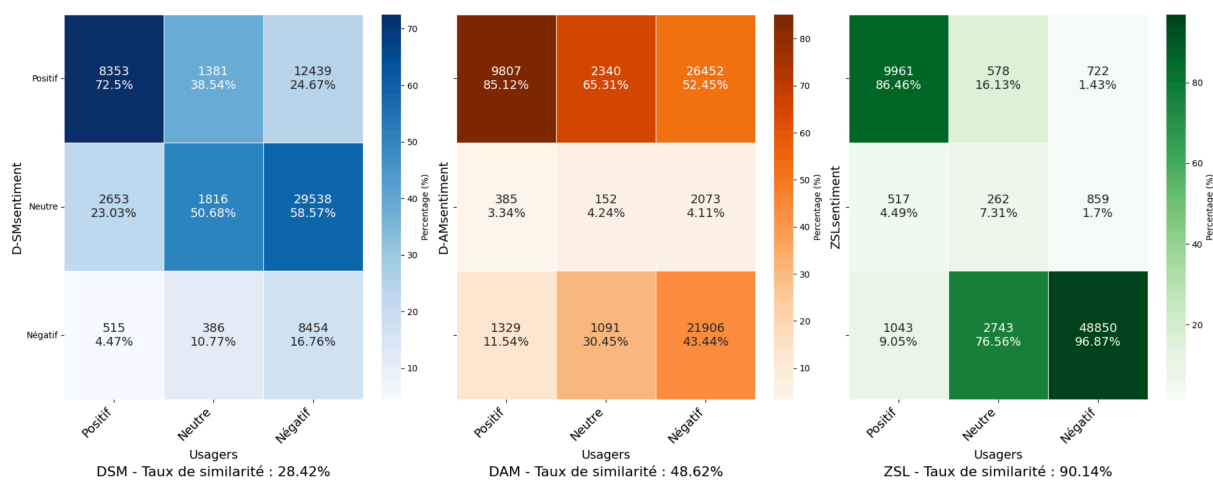
Figure 3.4 – Distribution des concordance entre la labellisation de chaque modèle et celle des usagers
