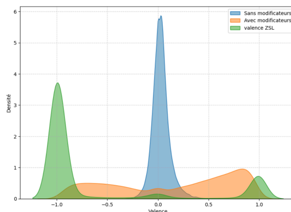
Figure 3.3 – Distribution des scores de valence par méthode.
